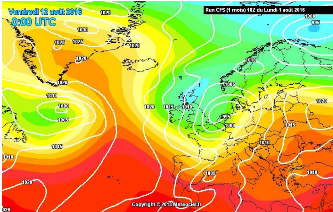
Géop. Z500 (dam) & pression au sol (+ 246h)
