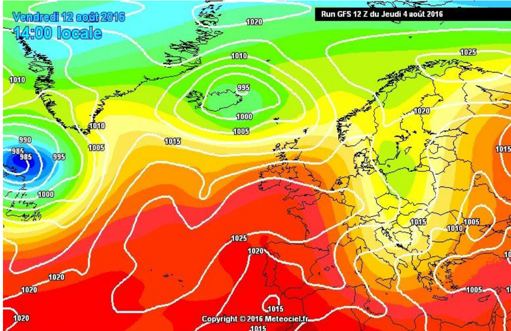
Géop. Z500 & pression au sol (+ 192h)
